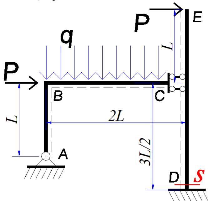
Fig. 1. Schema della struttura (dimensioni in metri) e geometria della sezione trasversale S-S
