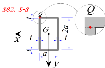
Fig. 1. Schema della struttura (dimensioni in metri) e geometria della sezione trasversale S-S
